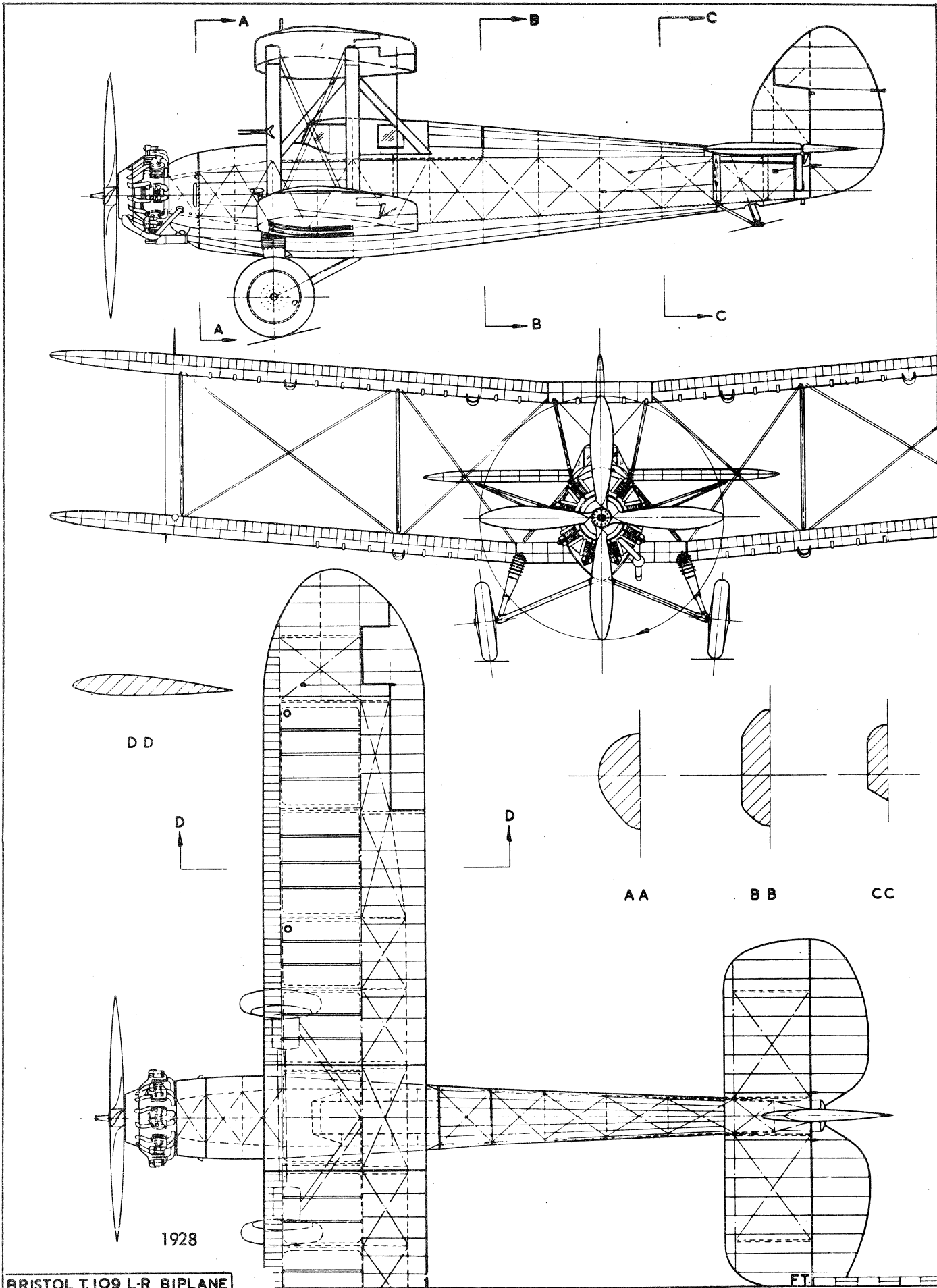
BRISTOL T.109 L-R BIPLANE
