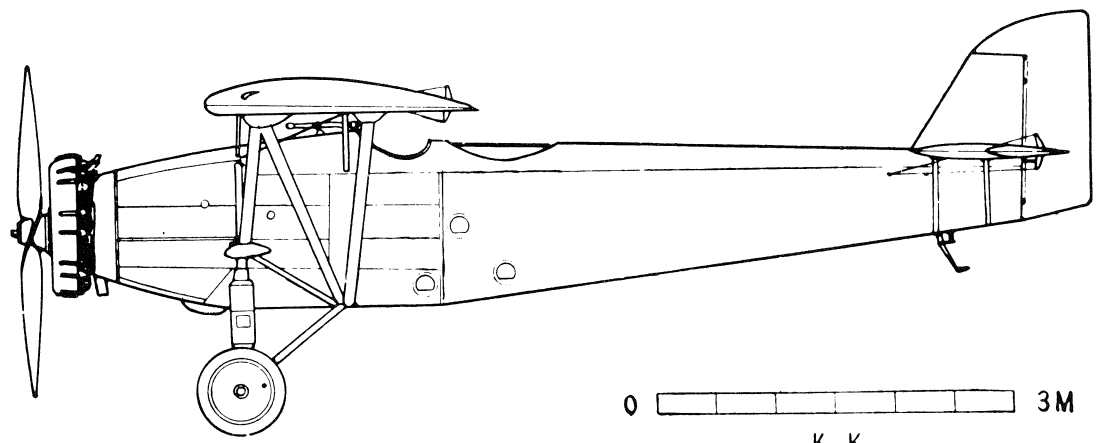
九二式偵察機 (2MR8) (第 1, 2 号機) ARMY TYPE 92 RECONNAISSANCE
