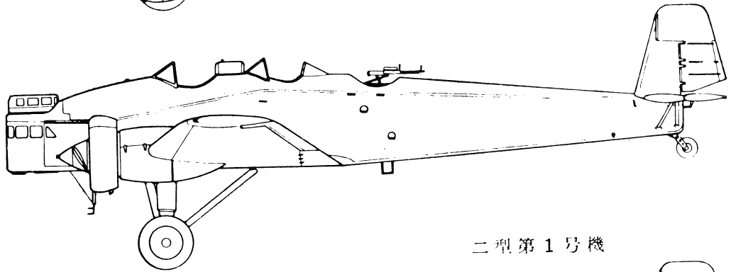
一型座席増設型
