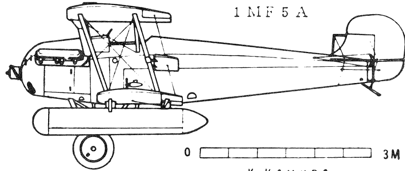
一〇式艦上戦闘機 NAVY TYPE 10 CARRIER FIGHTER
