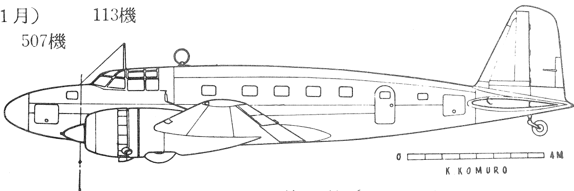
一〇〇式二型輸送機 (キ-57-II) ARMY TYPE 100 TRANSPORT - KI-57
