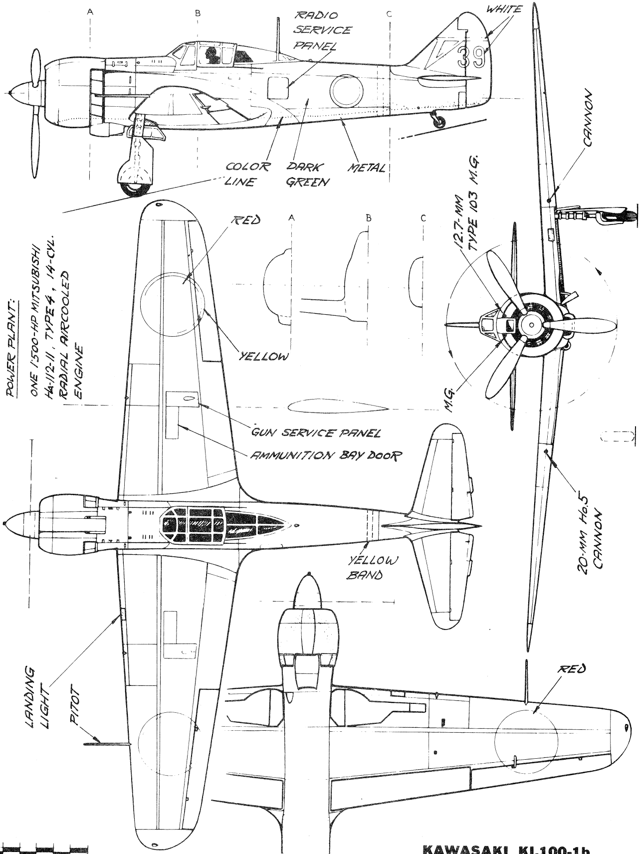
KAWASAKI KI.100-1b
