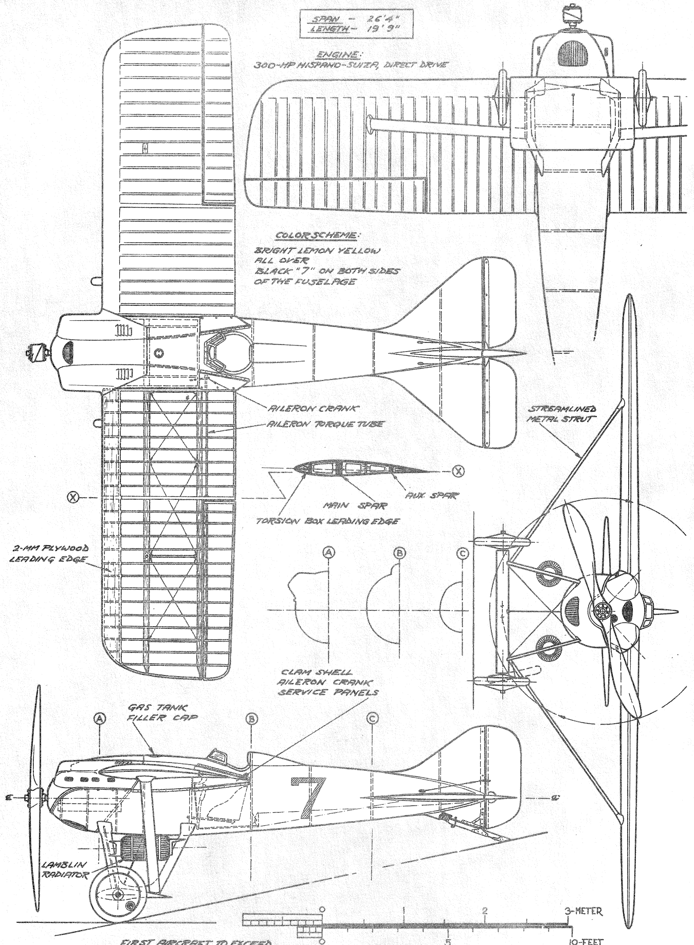
KARLSTROM: 1921 NIEUPORT SESQUIPLANE RACER
